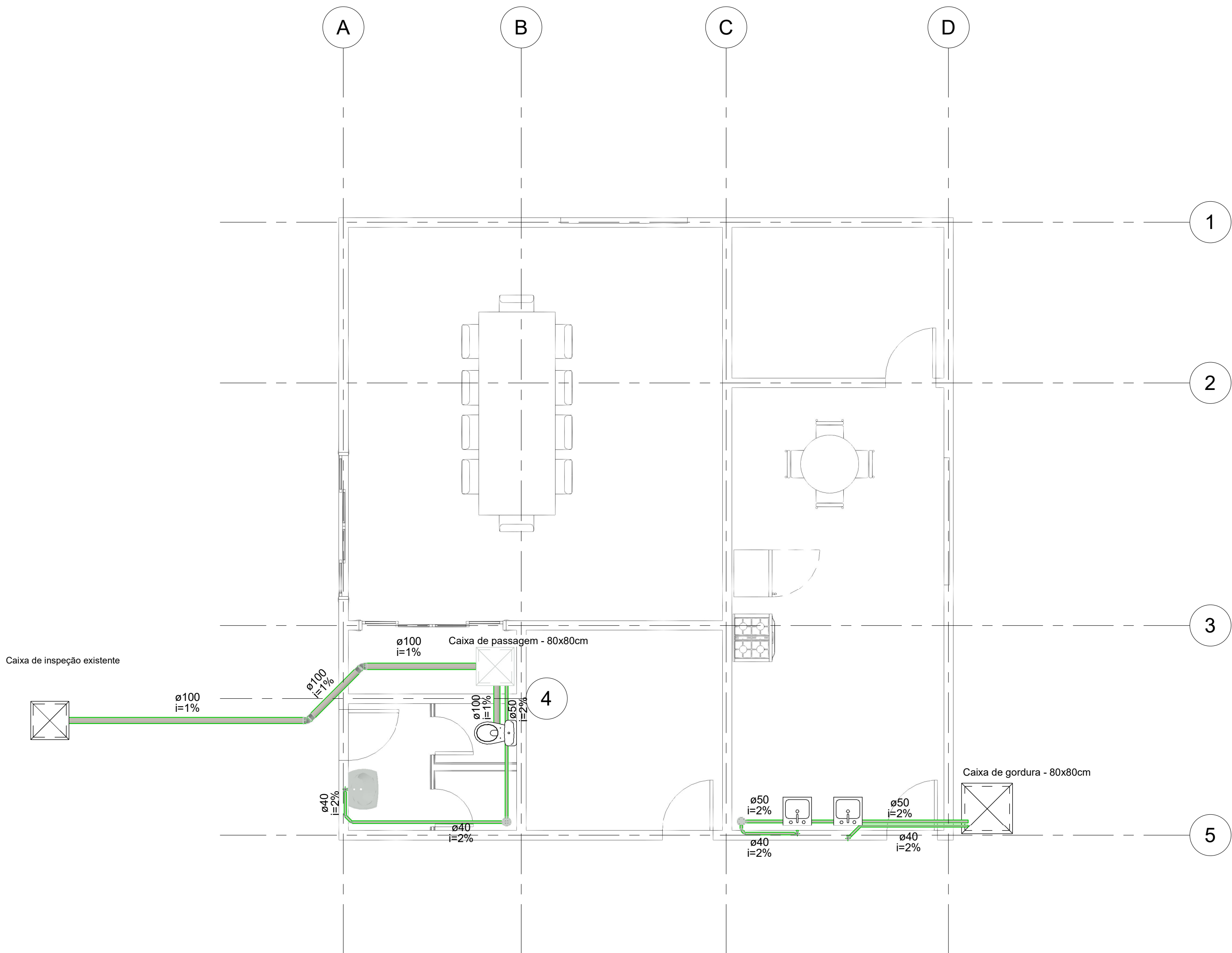
1 Sanitário - Banheiros 1 : 50
