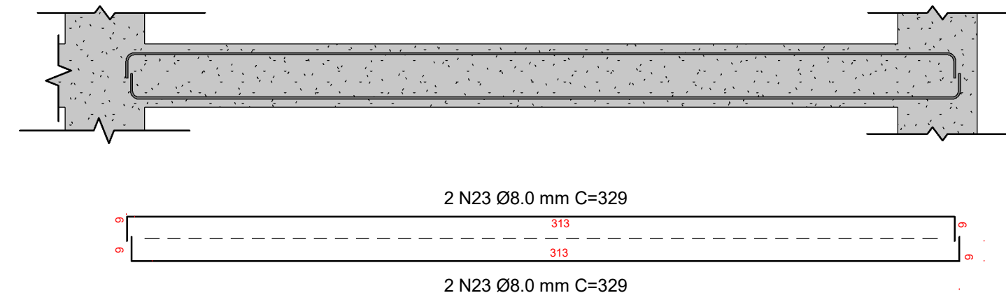
7 VIGA Baldrame 15 x 24 cm 1 : 20
