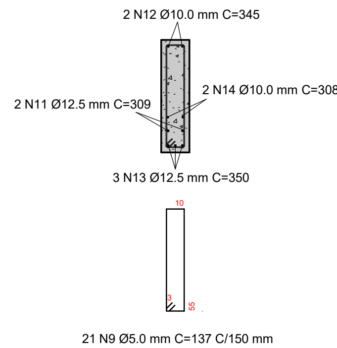
12 Estribos - Viga 15 x 60 cm 1 : 20
