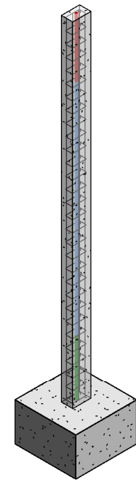
PESPECTIVA PILAR 15 x 30 cm
