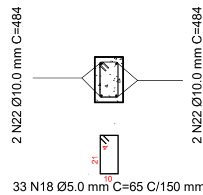
5 Estribos Pilar 15x26 cm 1 : 20
