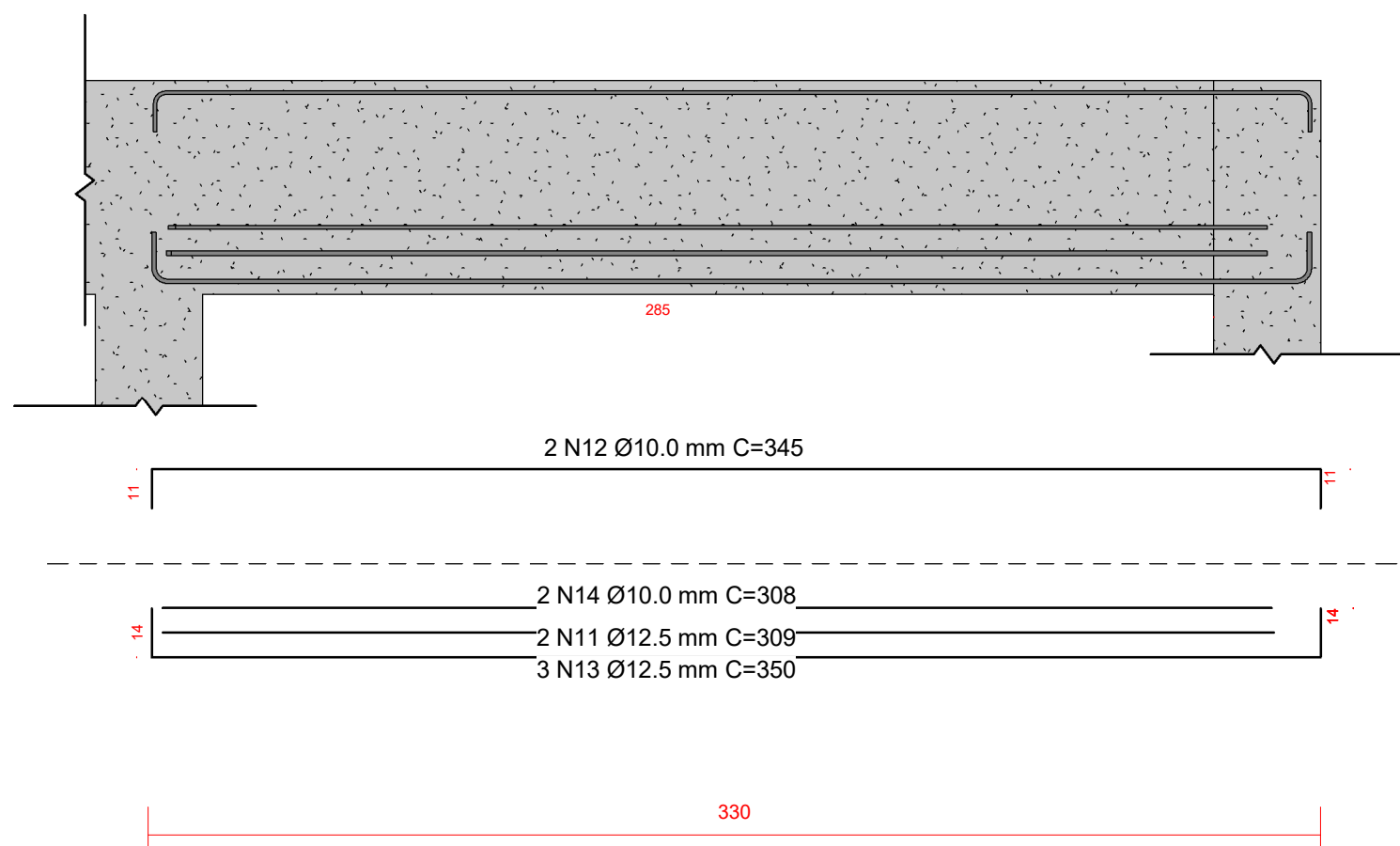
11 VIGA 15 x 60 cm 1 : 20
