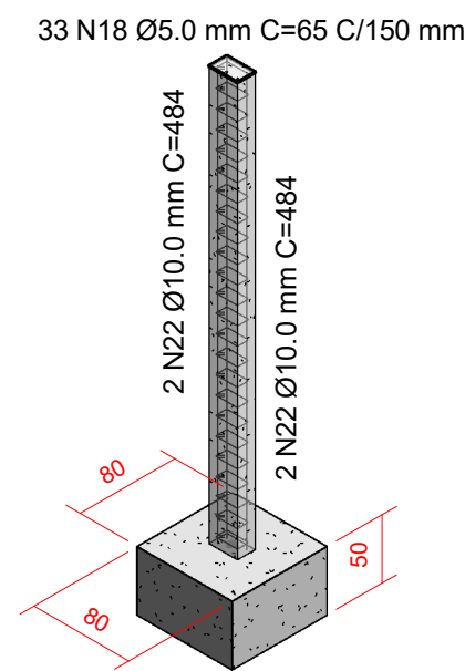
PESPECTIVA PILAR 15 x 26 cm
