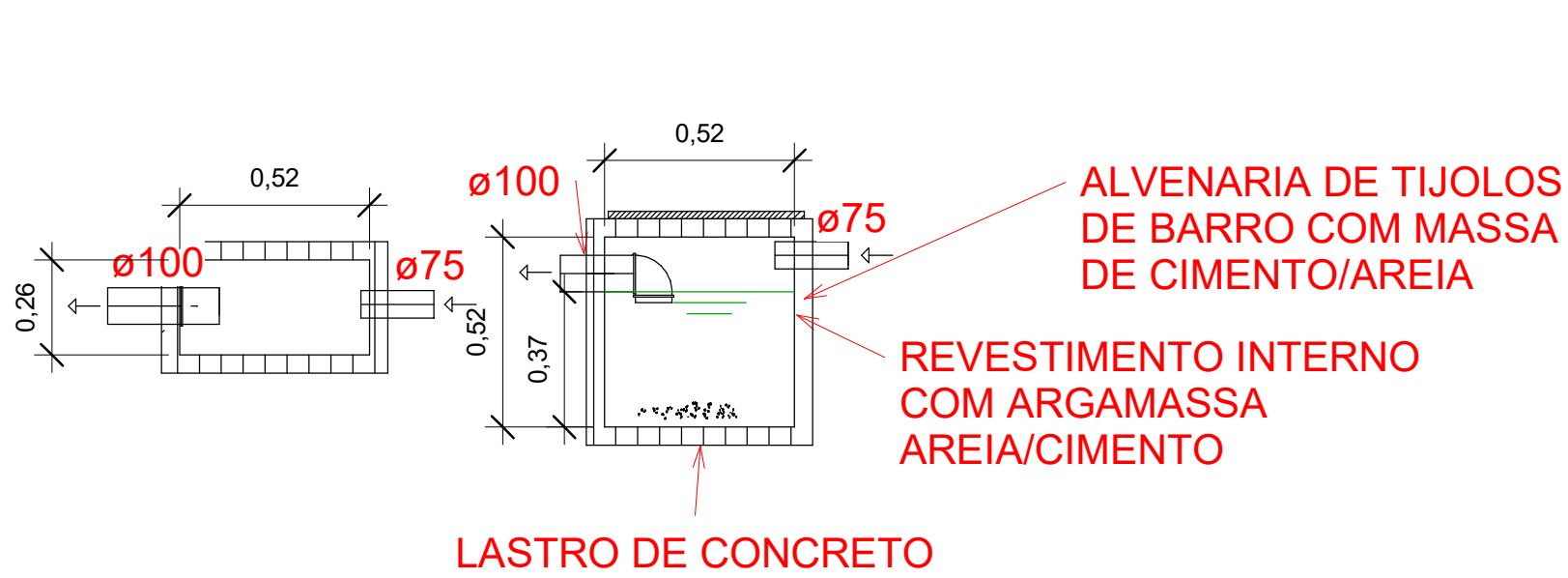
2 Caixa de gordura 1 : 20
