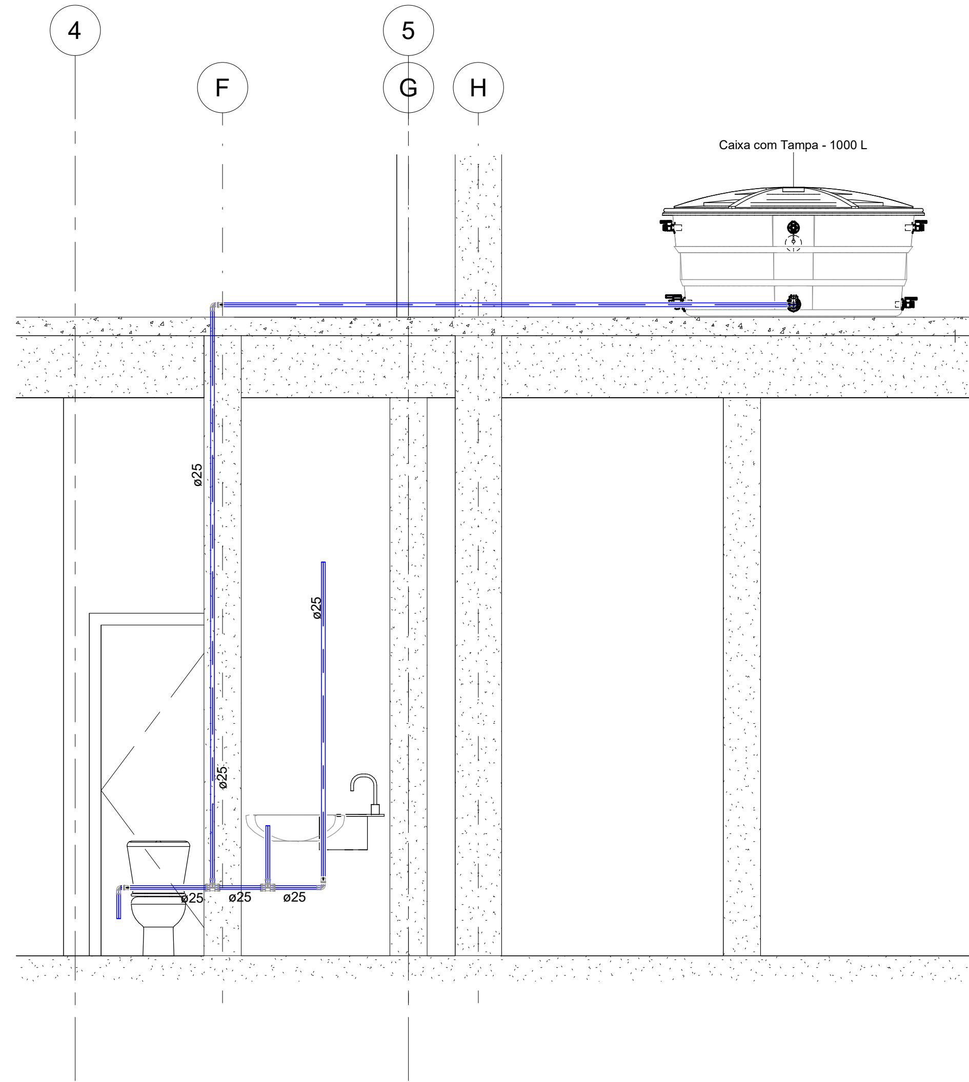
4 HID_CORTE A- BANHEIROS 1 : 25
