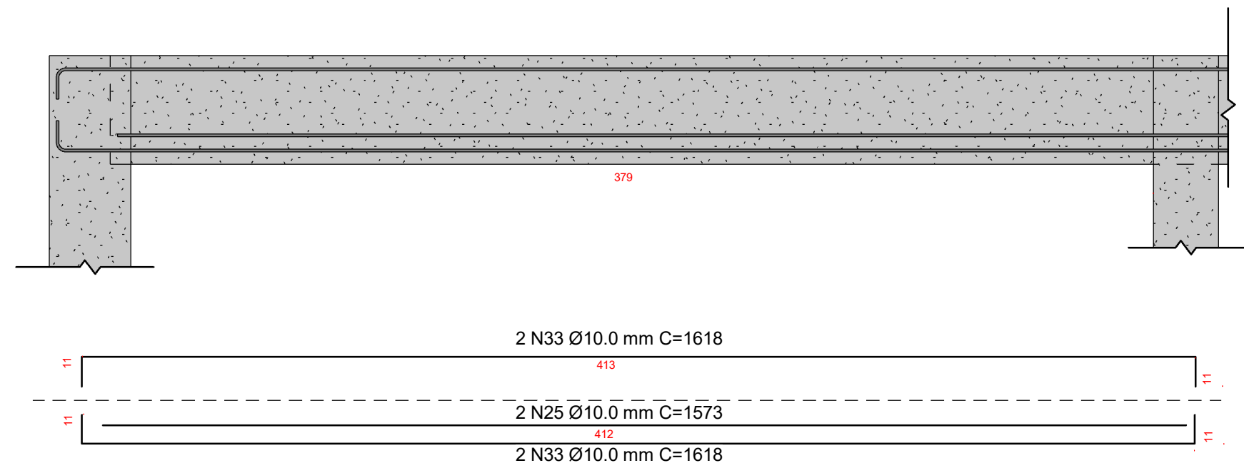
9 VIGA 15 x 40 cm 1 : 20
