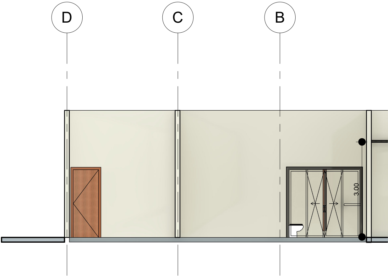
2 Corte A 1 : 75
