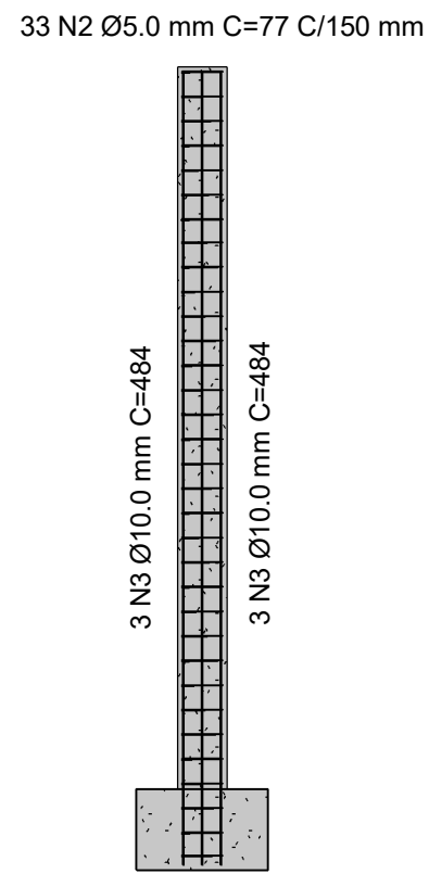
2 Pilar 15x30 cm 1 : 50
