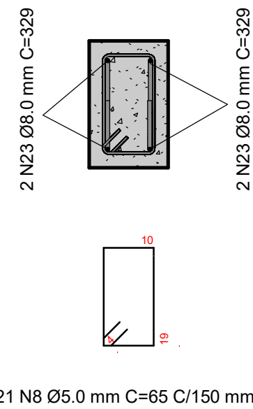
8 Estribos - Viga Baldrame 1 : 10
