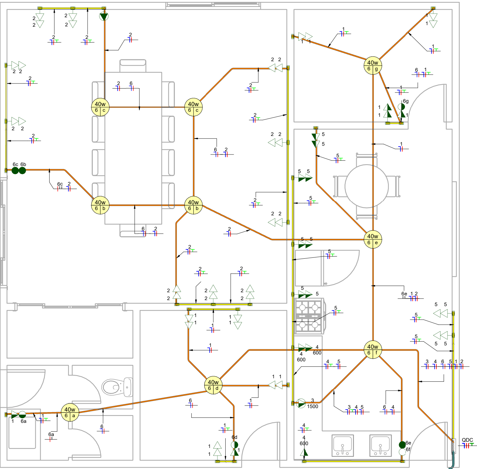
00 - Térreo
