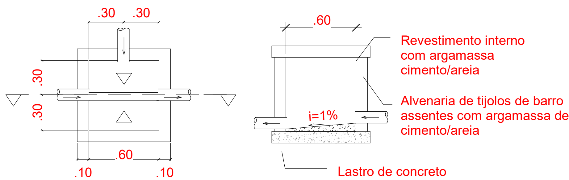
3 Caixa de inspeção 1 : 20
